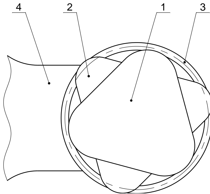
Рисунок 3 – Крепление абразивов
